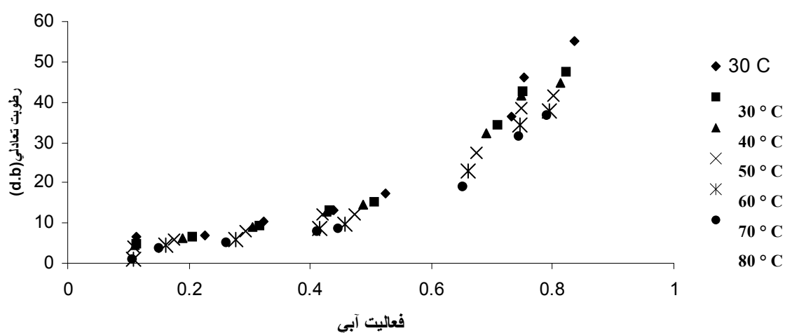
شکل ۲ - تأثیر دما بر رطوبت تعادلی کشمش بیدانه سفید در دماهای ۳۰، ۴۰، ۵۰، ۶۰، ۷۰ و ۸۰ درجه سانتی‌گراد Fig. 2. Effect of temperature on equilibrium moisture for Thompson seedless raisins from 30 to 80 °C
